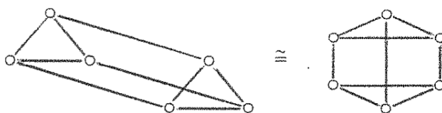
Fig. 4. K_3 \square K_2 \cong C_6^c .
