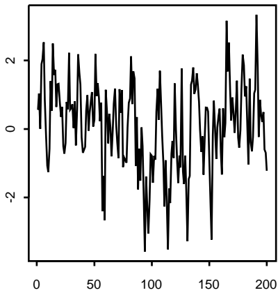
AR(1),phi=.5
